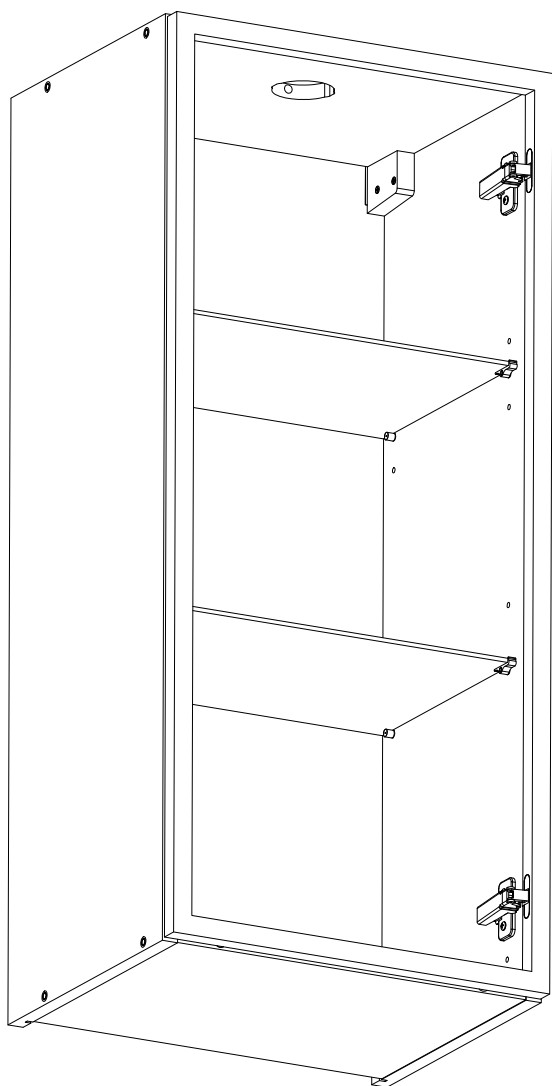
otworem oświetleniowym do wewnątrz szafki SZAFKA Z OŚWIETLENIEM WEWNĘTRZNYM
